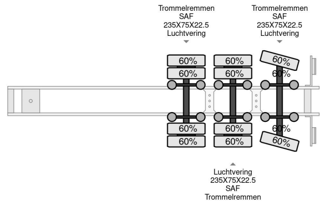
Bodex 3 AXEL TRUCKTRANSPORTER
