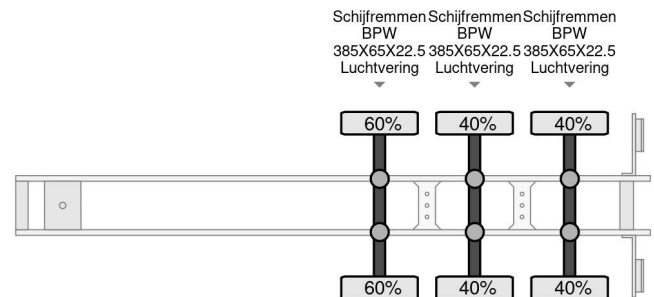
Lecitrailer MET HIAB R165 F3
