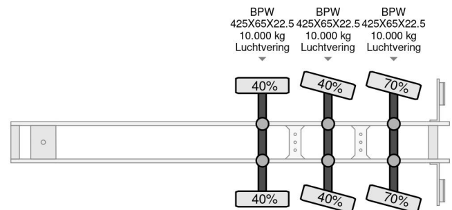
PACTON TRAILERS HIAB R220-F3+K MET ROTATOR EN P...
