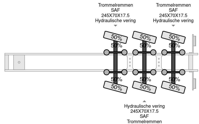
Faymonville MEGAMAX TL STBZ-3VA 4,5 M EXTENDABLE
