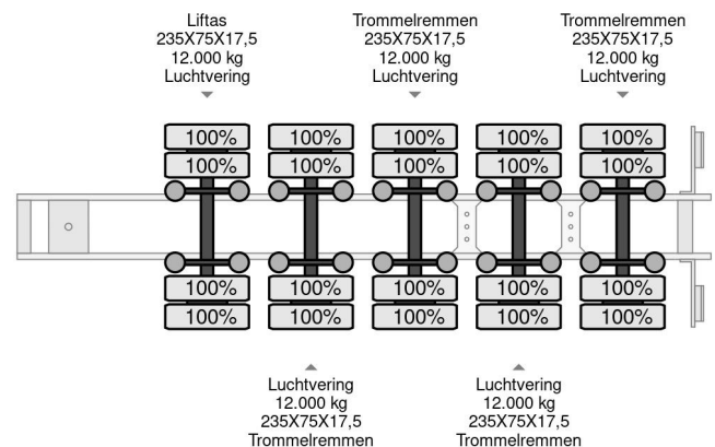
Scorpion NEW 5 AXEL 78 TON
