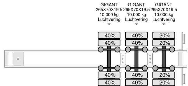
Diversen NC 3 AXEL 7,4 METER EXTENDABLE
