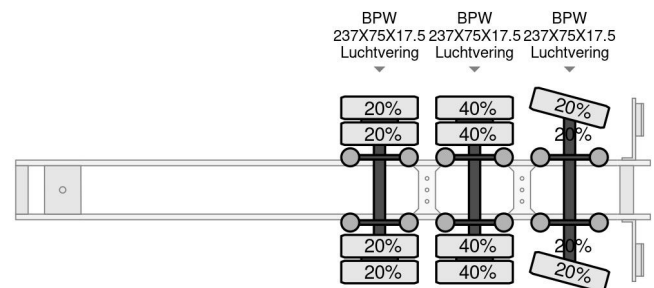
KELBERG E48-3 - BED 5,50 METER EXTENDABLE + HYD...
