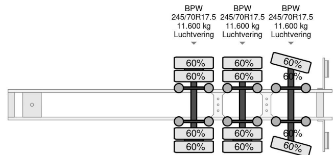
Goldhofer STN-L 3-38/80A - BED: 8,75 + 5,75 METER
