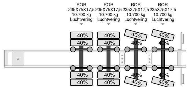
Kässbohrer 4 AXLE LAST 2 STEERING, EXTENDABLE
