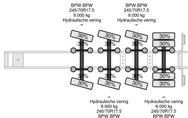
Nootboom MCO-58-04V - 4 AXLE BPW + 2X EXTENDABLE
