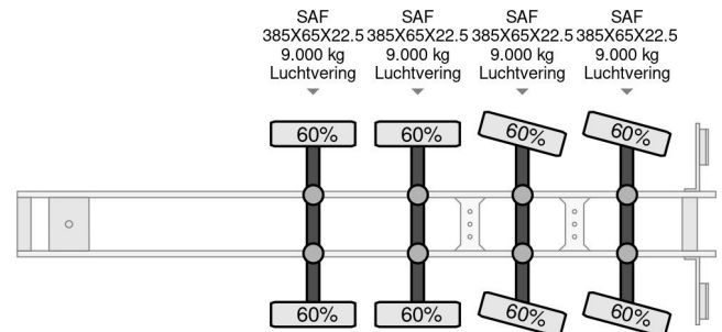
Pacton HIAB ROLLER 220 F5, 4 ASSIGE, 2 LIFT + 2 STUUR...
