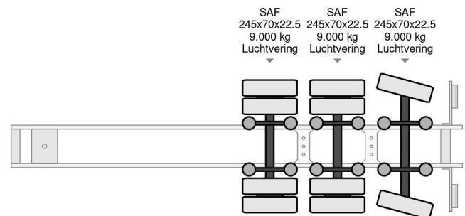
Nootboom OSDS-48-03V LAST AXLE STEERING, 6,8 M E...
