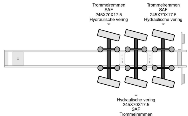
Nootboom EURO 54-03 3 AXLE STEERING 5,3 METER EX...
