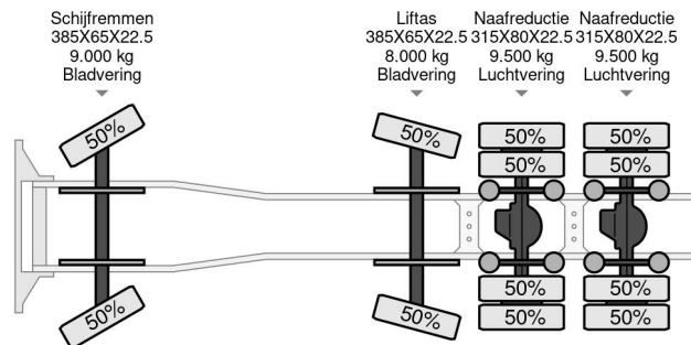
DAF XF 530 8X4 140 TON 384000 KM
