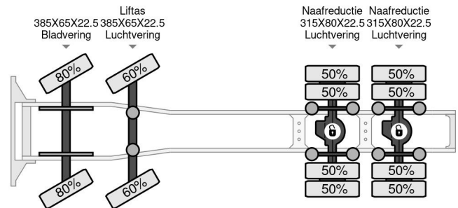
MAN TGX 41.540 8X4 180 TON RETARDER
