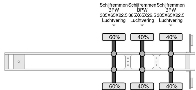
Lecitrailer MET HIAB R165 F3
