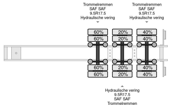
Nootboom OSD-44-VV + 3 AXLE SAF + 5 METER EXTEND...
