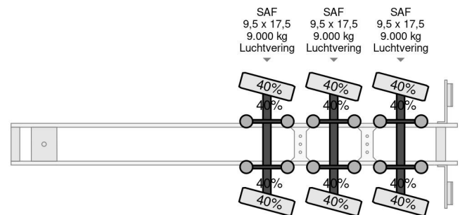
Nooteboom OSDBAZ-41-VV 3,3 METER EXTENDABLE, 3 A...
