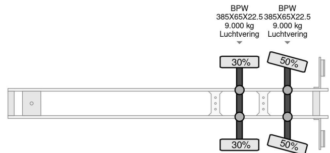
VAN HOOL LAST AXEL STEERING, LIFT 2000KG
