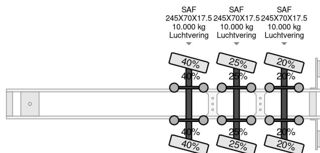
Broshuis 3 X EXTENDABLE TOTALE 42 M + EXTENSION T...
