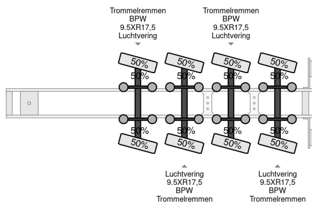
Goldhofer 4 AXEL STEERING
