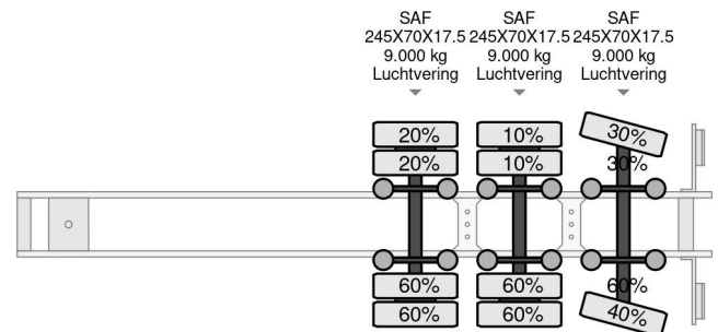
Nooteboom OSDS 48-03V 6,8 M EXTANDABLE
